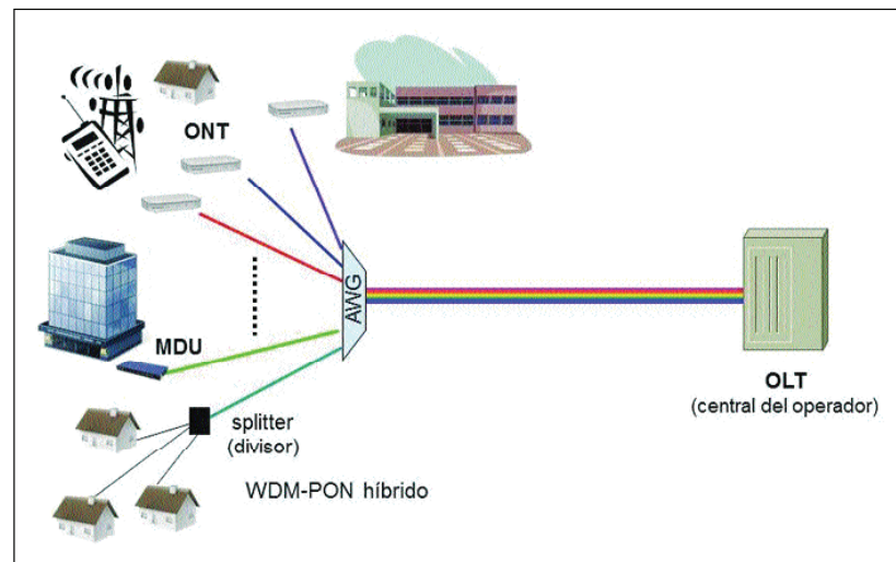
Figura 1: Arquitectura de WDM-PON.
